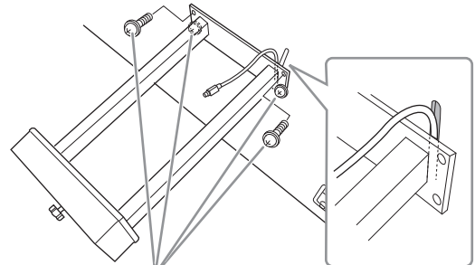
Tornillos de fijación de 6 x 20 mm
